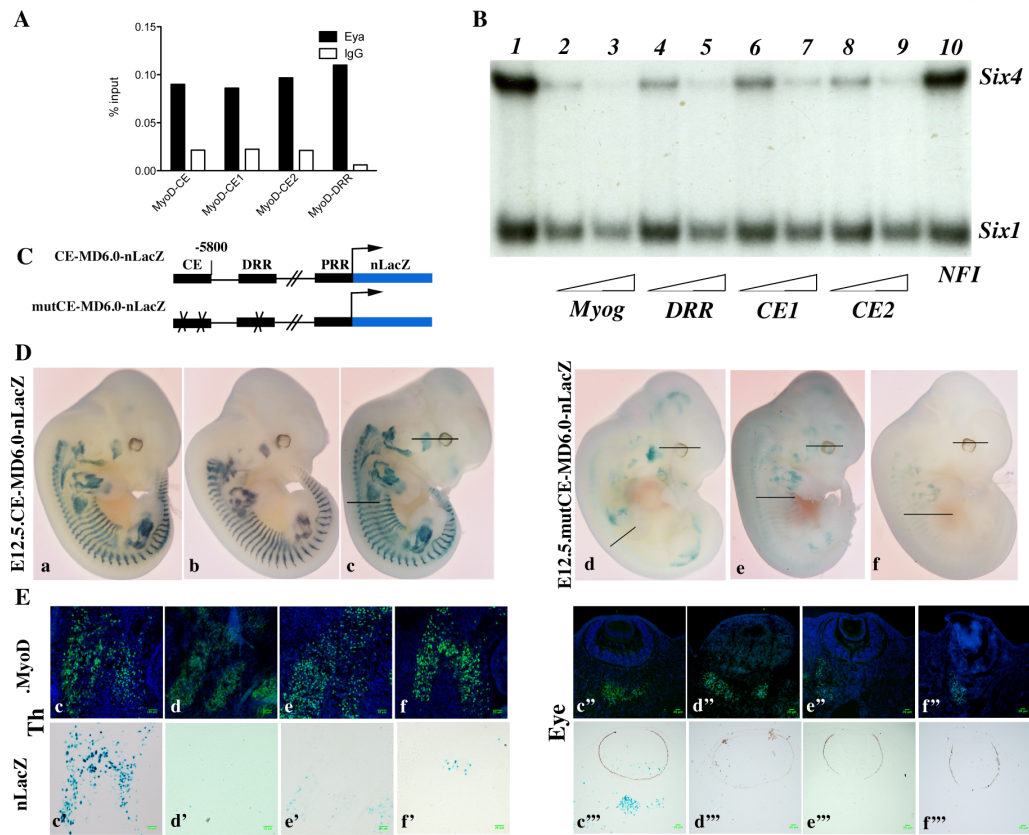
FIGURE 5.8 – Validation des sites MEF3 prédits dans les éléments régulateurs de Myod1 . Figure présentée dans l'article Relaix et al. (2013) . Plus de détails sont donnés dans le texte principal. (A) Expérience de ChIP montrant que les protéines Eya, cofacteurs de Six1 et Six4, sont recrutées au niveau du CE et du DRR. (B) Expériences de retard sur gel (EMSA) montrant que Six1 et Six4 interagissent avec les sites prédits sur les enhancers. (C) Schéma des transgènes wild-type et mutés en sites MEF3. (D) Coloration au X-Gal d'embryons à E12.5 porteurs de transgènes des séquences wild-type (a, b, c) et mutantes (d, e, f), montrant l'abolition de l'expression du gène rapporteur lorsque les sites MEF3 sont mutés. (E) Analyse de l'expression de MyoD par immunohistochimie et du rapporteur LacZ par coloration X-Gal dans les coupes indiquées par un trait noir chez les embryons c, d, e et f au niveau du thorax (Th) et des yeux (Eye). On note l'absence d'expression du transgène muté dans les cellules exprimant MyoD.
