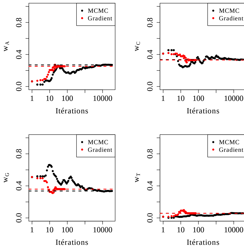
FIGURE 3.5 – Comparaison des approches par MCMC et par descente de gradient.
