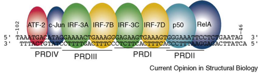
FIGURE 1.17 – L'enhanceosome de l'interferon- \beta .
