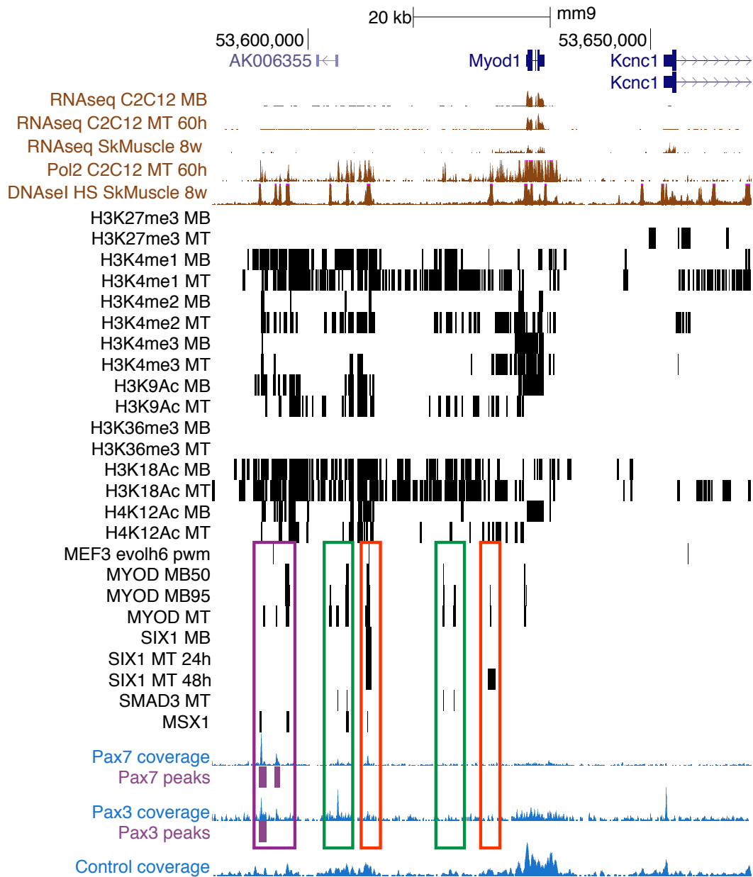
FIGURE 5.6 – Visualisation de données musculaires sur UCSC.
