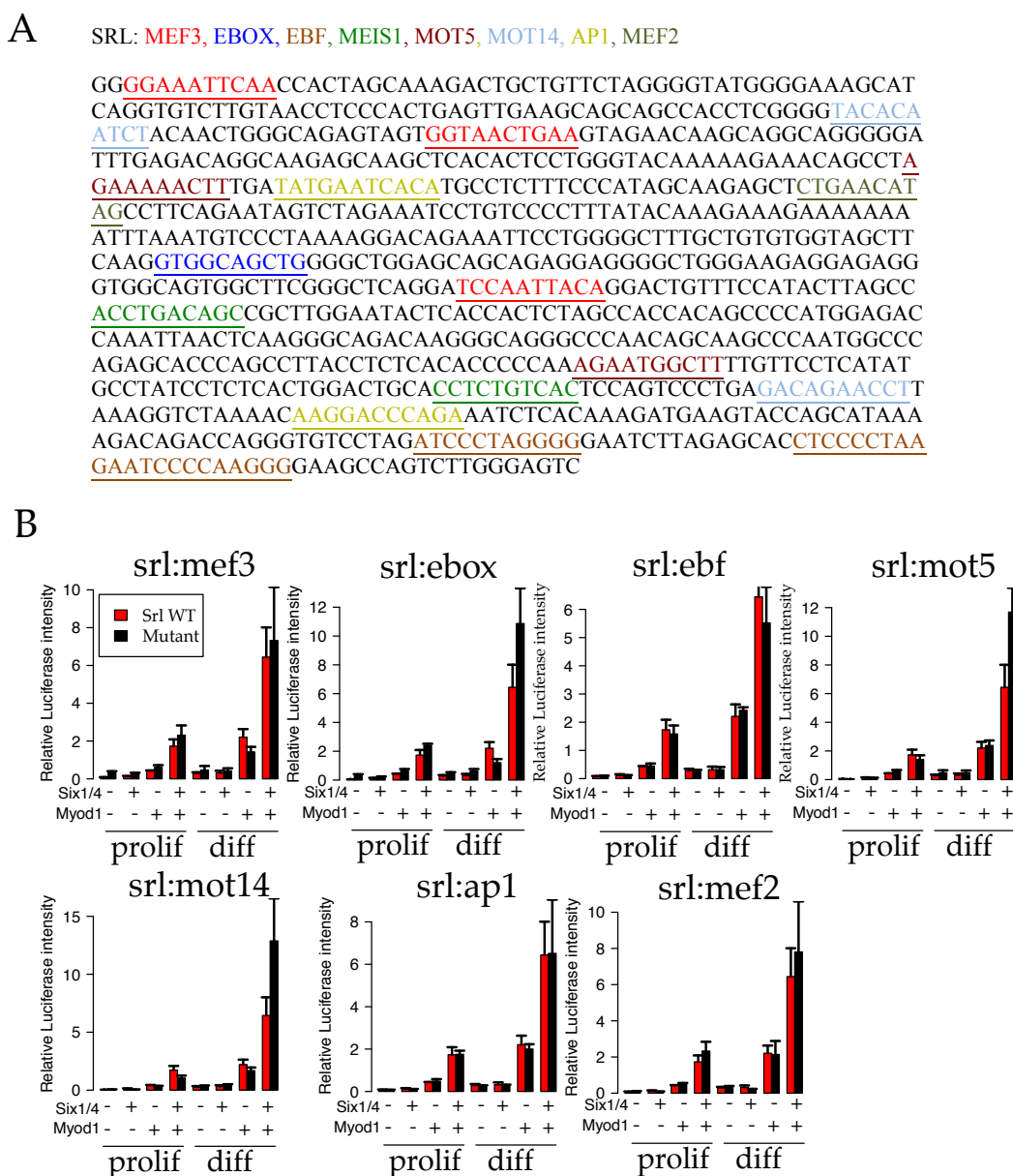
FIGURE 5.19 – Mutagenèse systématique des sites prédits sur l'enhancer de Srl .
