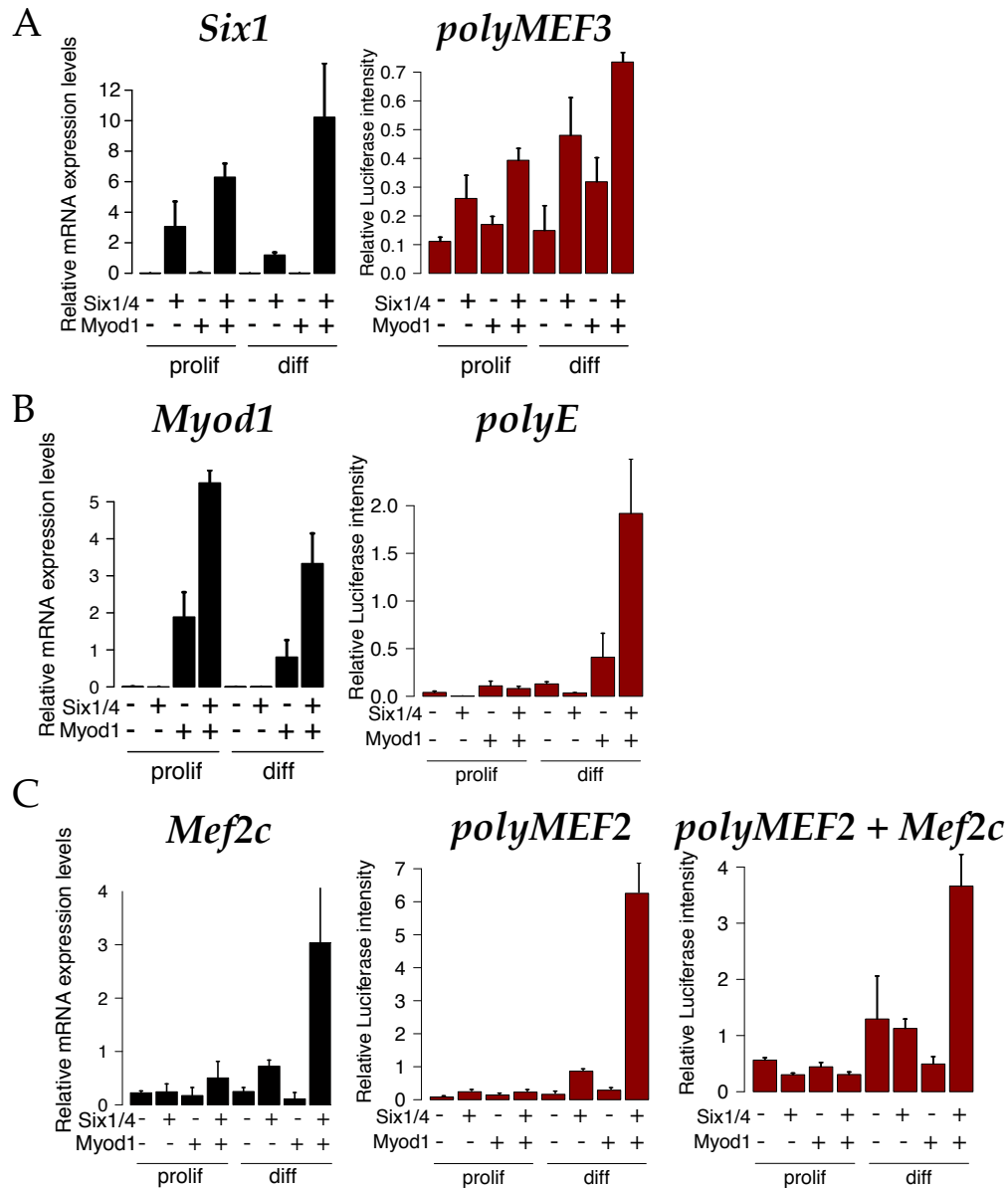
FIGURE 5.21 – Expression Luciférase de multimères synthétiques de sites de fixation. Diverses expériences de Luciférase sont montrées pour des enhancers synthétiques contenant des multimères de sites de fixation, ainsi que l'expression du TF correspondant. (A) Séquence polyMEF3 contenant 6 sites MEF3. (B) Séquence polyE contenant 4 E-Box. (C) Séquence polyMEF2. Dans ce dernier cas, l'un des deux multimères a été co-transfecté avec un vecteur d'expression Mef2c
