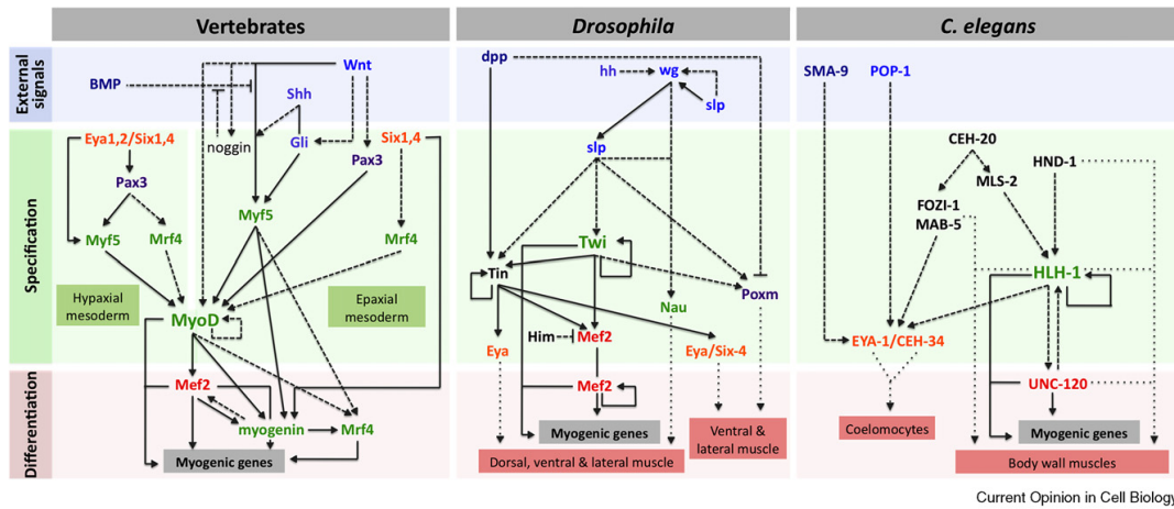
FIGURE 1.8 – Évolution du réseau transcriptionnel : l'exemple de la régulation myogénique..
