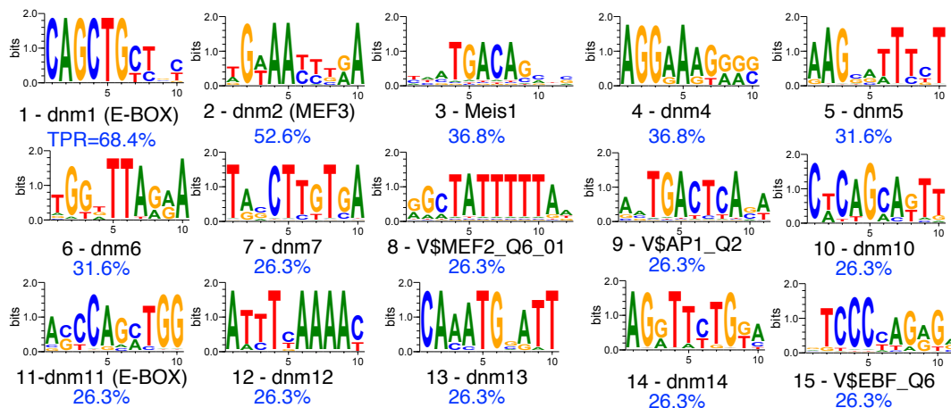
FIGURE 5.18 – Motifs sur-représentés sur les enhancers synergiques.
