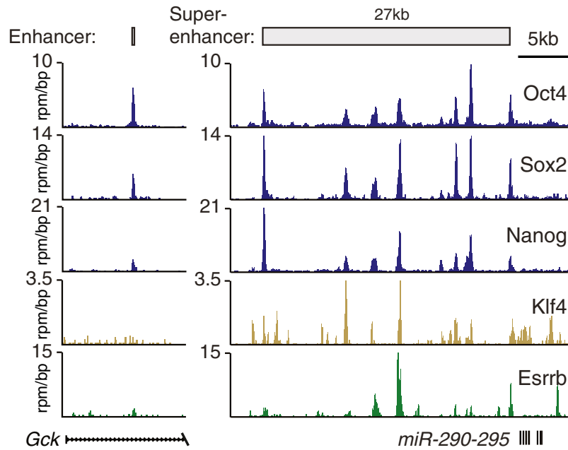
FIGURE 1.21 – De l’enhancer au super-enhancer.
