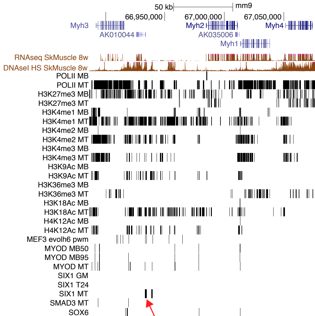
FIGURE 5.9 – Visualisation du locus des myosines sur UCSC.
