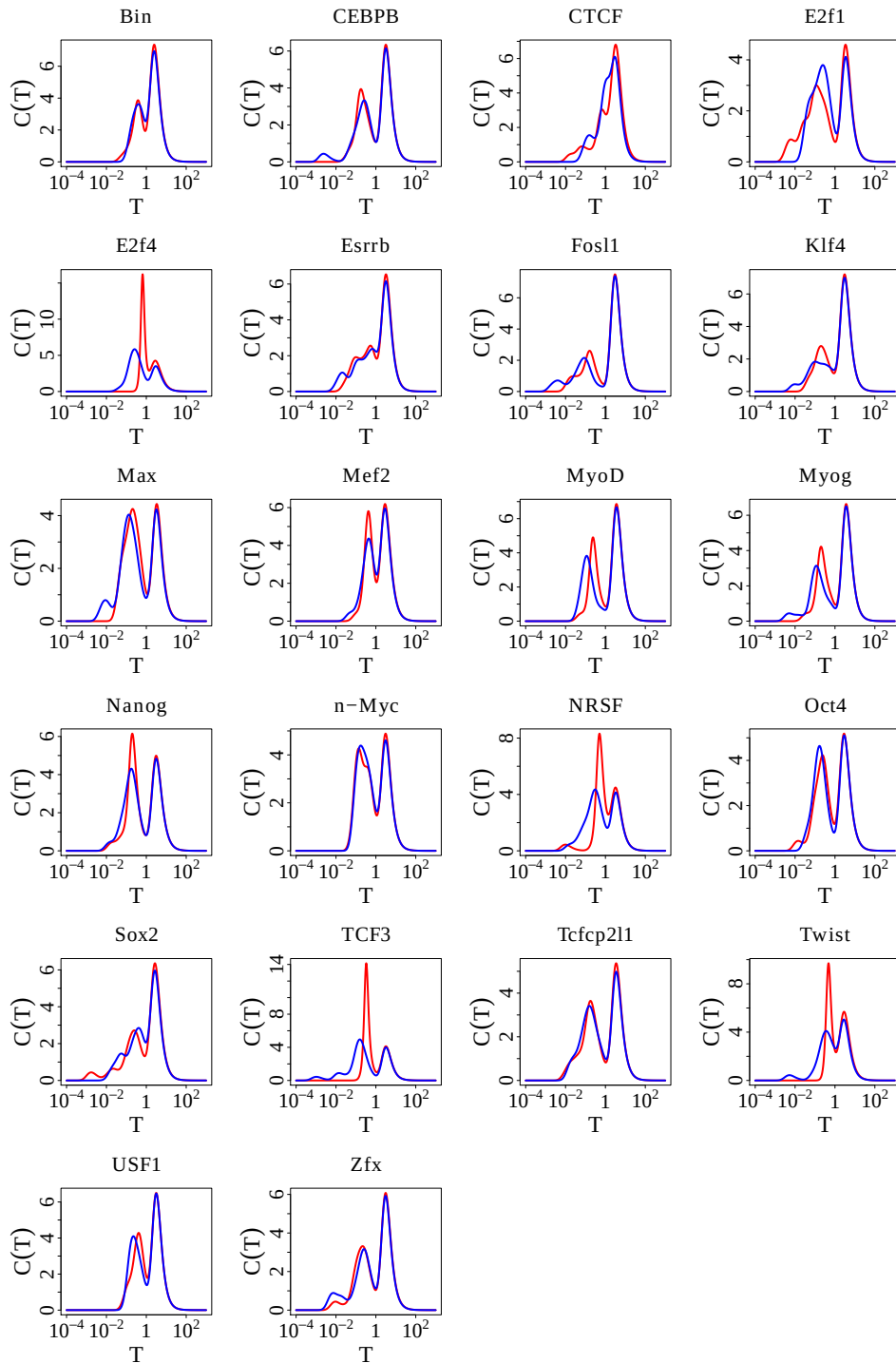
FIGURE 2.3 – Chaleur spécifique pour différents TFs.
