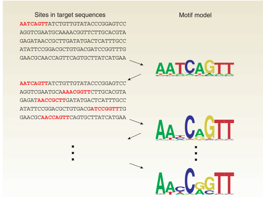
FIGURE 3.1 – Illustration de l’approche Espérance-Maximisation.
