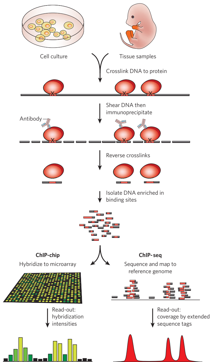
FIGURE 1.11 – Étapes d’une expérience de ChIP-on-chip et ChIP-seq.
