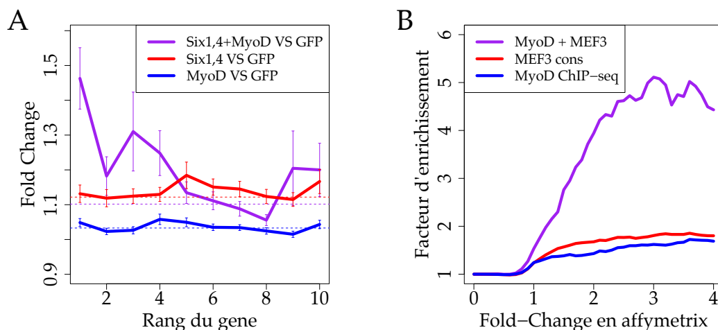
FIGURE 5.13 – Rôle des enhancers putatifs MyoD+MEF3 dans la synergie Six+MyoD.
