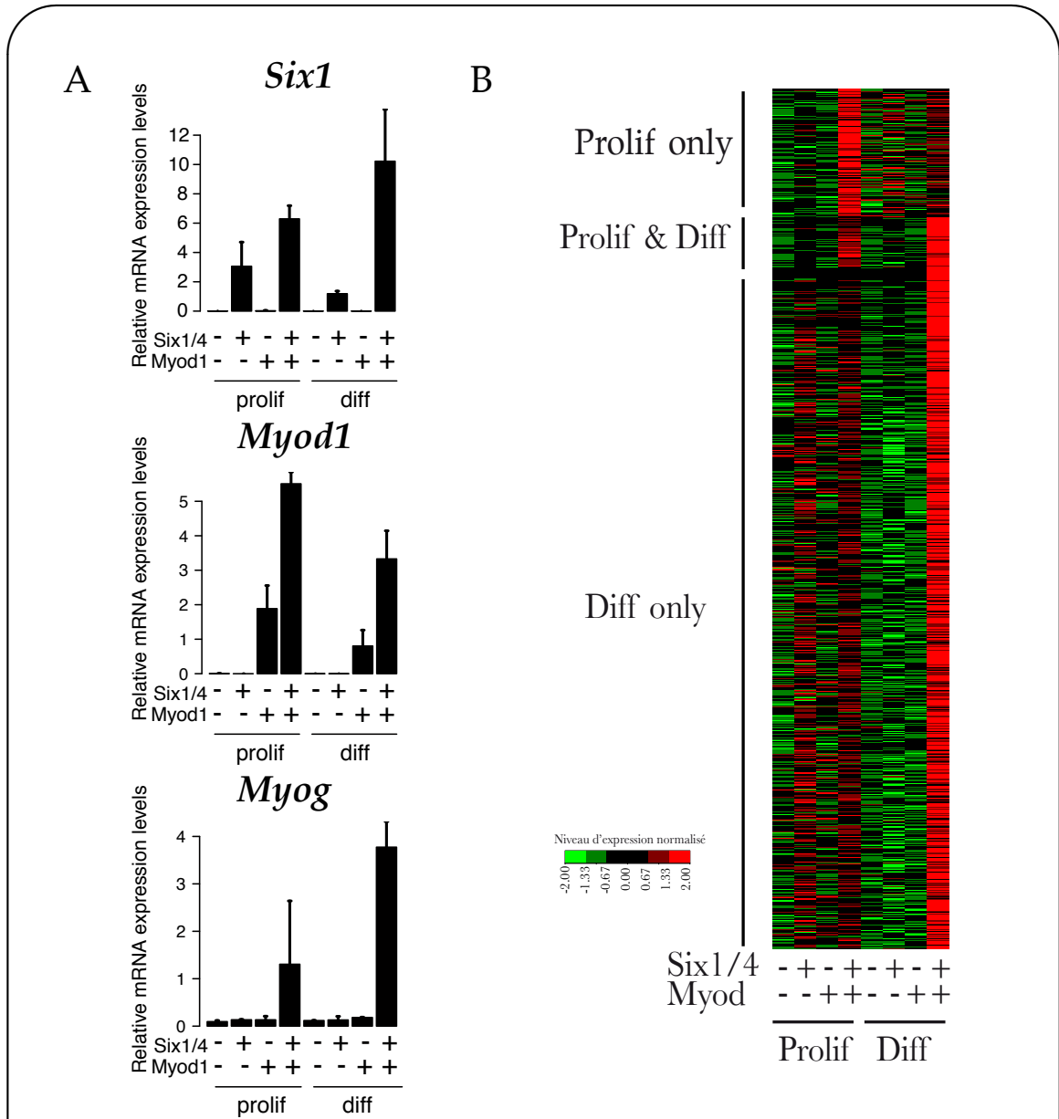
FIGURE 5.11 – Données d'expression des gènes activés par la synergie Six+MyoD.
