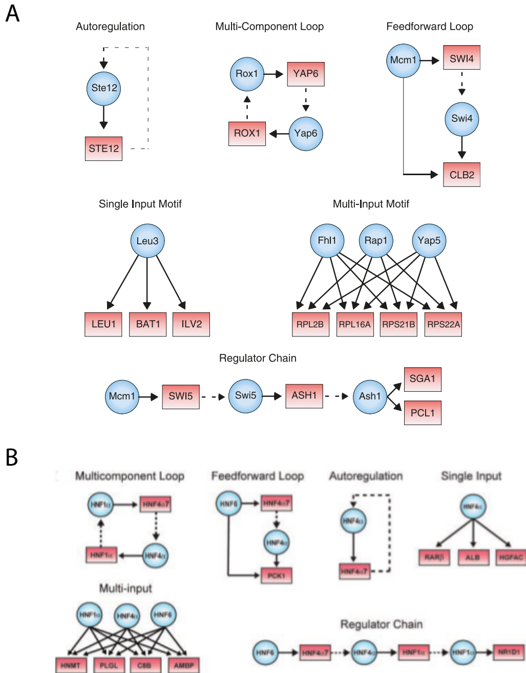
FIGURE 1.7 – Exemples de motifs dans les réseaux de régulation génétique.
