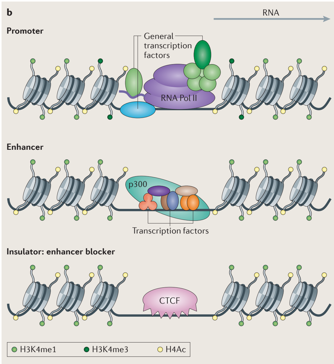
FIGURE 1.14 – Les différents types de CRMs et leurs marques épigénétiques.
