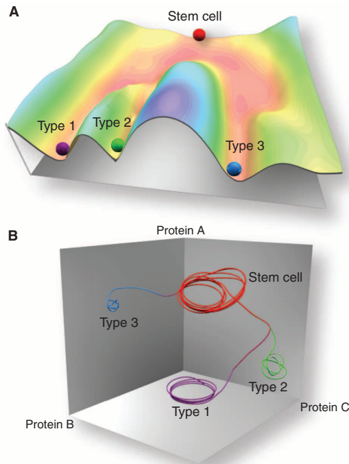
FIGURE 1.1 – Le paysage de la différenciation cellulaire.
