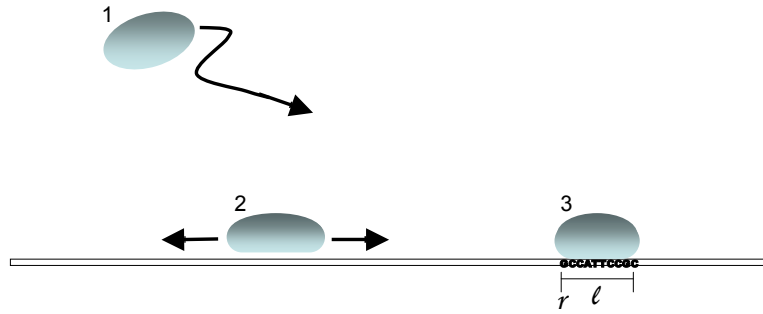
FIGURE 1.9 – Différents états du facteur de transcription. Figure tirée de (Lässig, 2007). Lors de sa recherche de site de fixation, le TF peut se trouver dans trois états distincts : (1) un état libre de diffusion tridimensionnelle, (2) un état de diffusion unidimensionnelle sur l'ADN par fixation non spécifique, et (3) un état de fixation spécifique. L'énergie de fixation dépend du site de fixation, de taille l et de coordonnée r .
