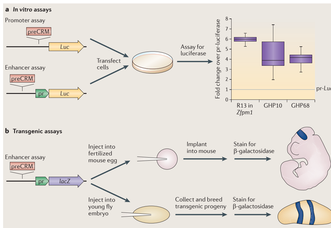
FIGURE 1.23 – Méthodes de validation des CRMs par transfection et transgénèse.
