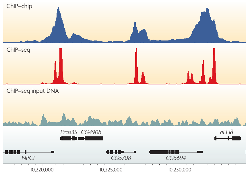
FIGURE 1.12 – Résolution des expériences ChIP-on-chip et ChIP-seq. Figure tirée de (Park, 2009), montrant les profils de fixation de la protéine Chromator générés à partir d’expériences de ChIP-on-chip (intensité relative par rapport au contrôle, bleu) et de ChIP-seq (densité de séquences, rouge) dans la lignée cellulaire S2 de Drosophila melanogaster . On peut noter la plus grande résolution de l’expérience ChIP-seq pour déterminer les sites de liaison. L’ADN utilisé en input de l’expérience de ChIP-seq et servant de contrôle est montré en gris, et les gènes du locus indiqués en noir.
