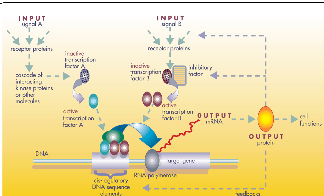
FIGURE 1.5 – Un réseau de régulation génétique type.
